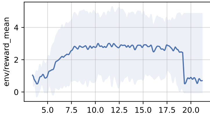
sentiment-analysis:cerebras/Cerebras-GPT-6.7B
